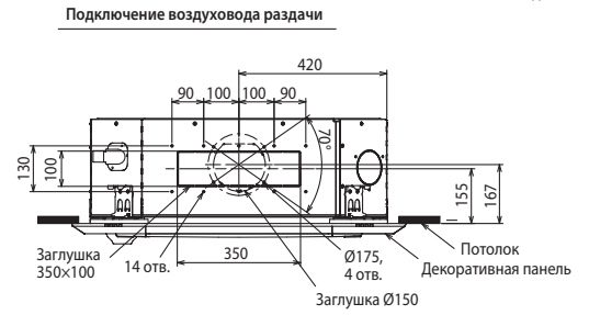
Подключение приточного воздухопровода
